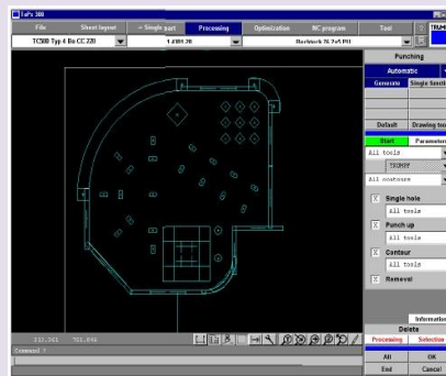
Slika 12. Procesiranje CNC-programa
