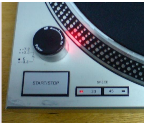
Slika 1. Stroboskop na gramofonu
